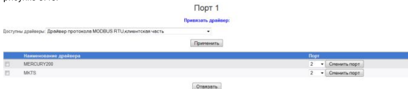
Рисунок 3.46 – Настройка параметров последовательных интерфейсов
